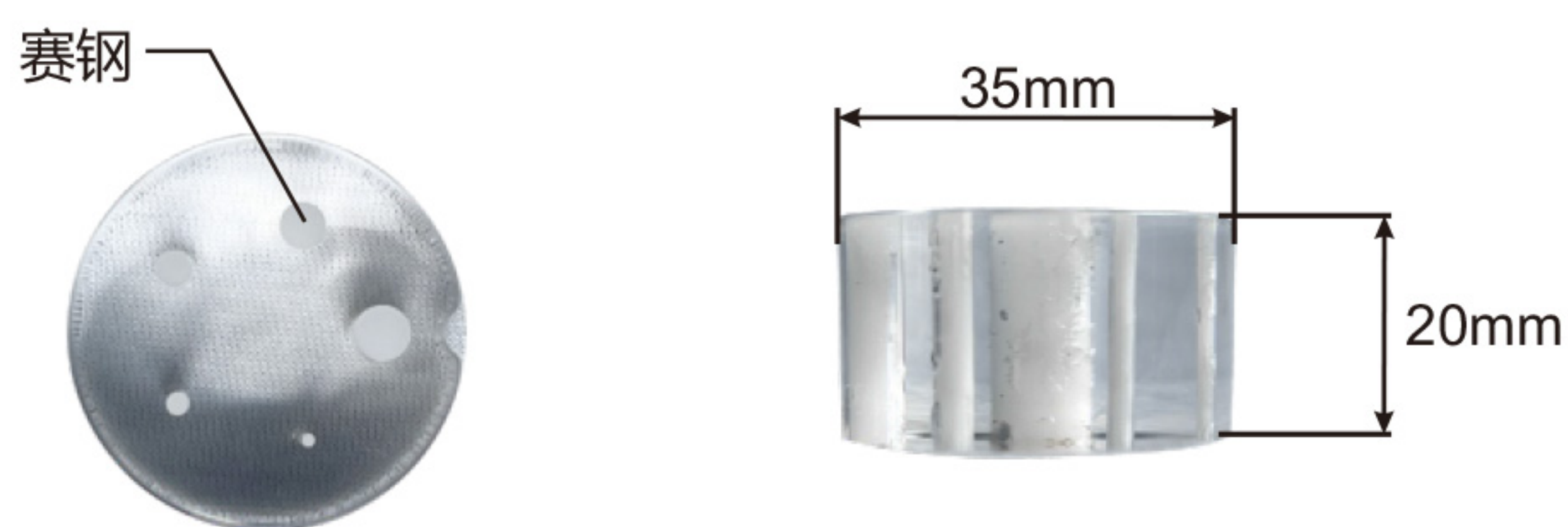
图 A.2 高对比度分辨力测试模块
