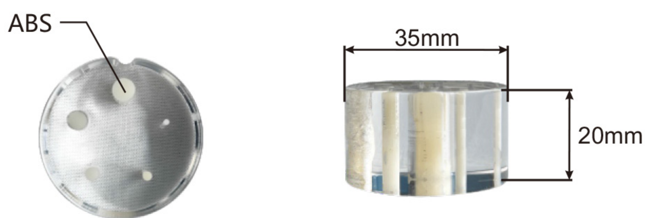
图 A.3 低对比度分辨力测试模块
